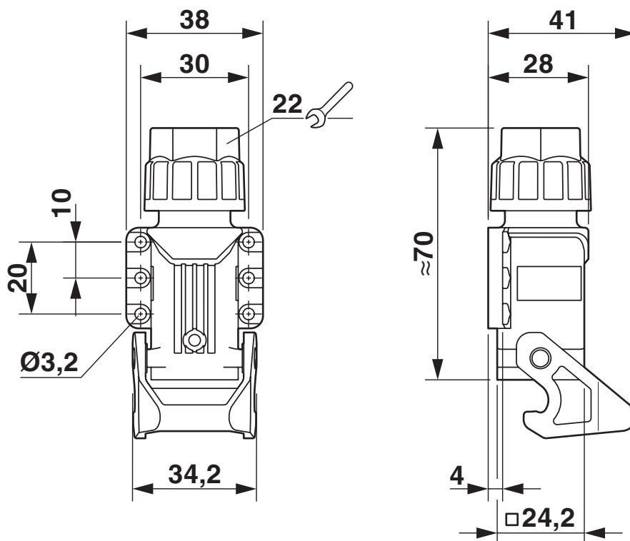
Dessin coté
