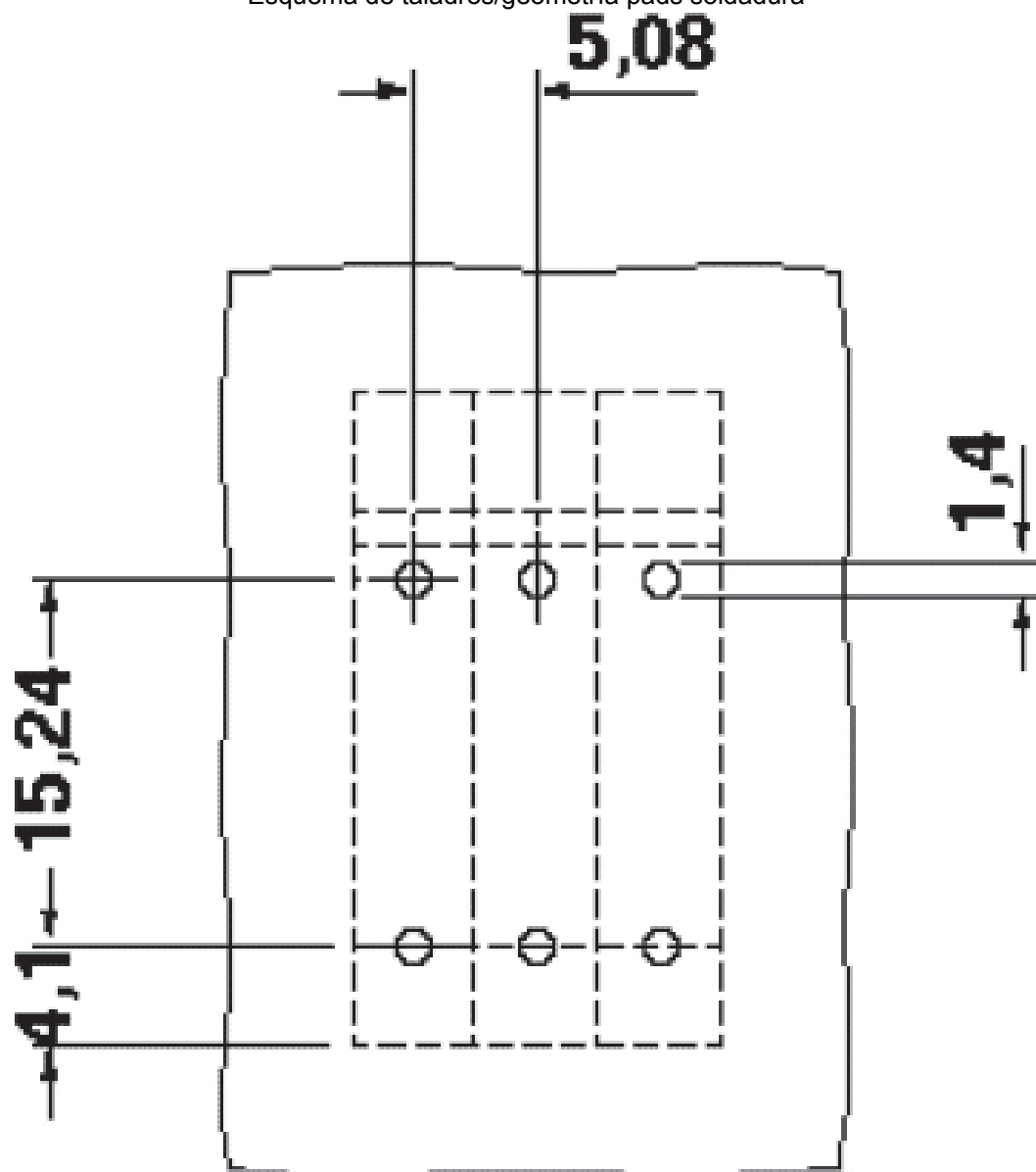
Esquema de taladros/geometría pads soldadura
