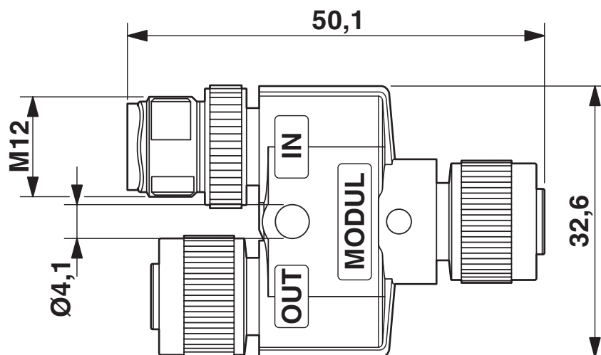
Connecteur mâle M12x1, répartiteur en Y
