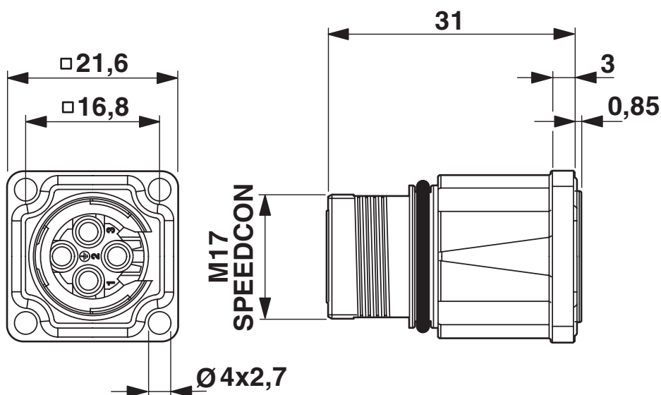
Dessin coté
