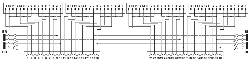
Schaltplan
