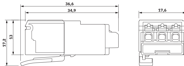
Maßzeichnung
