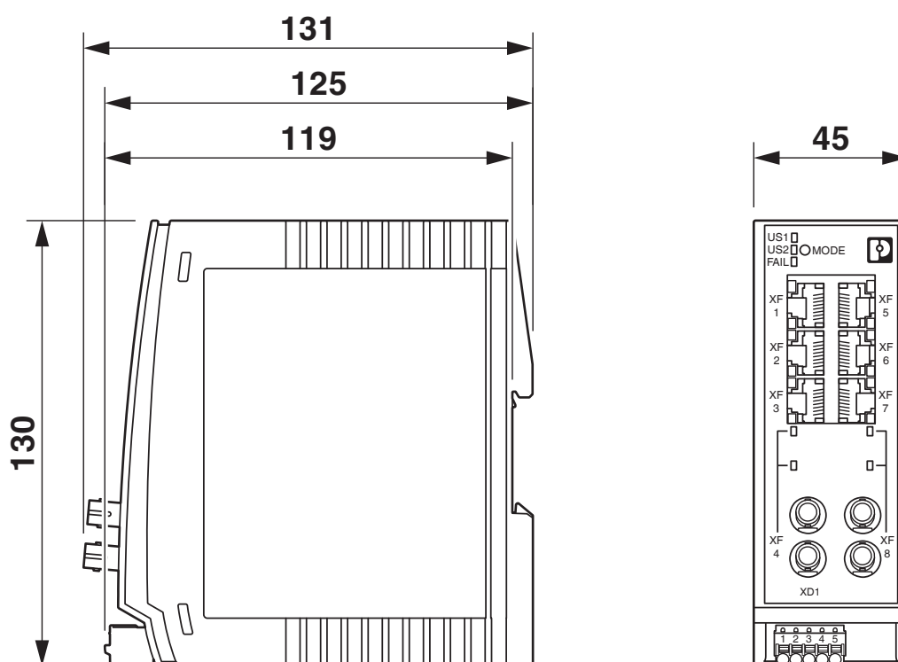
Dessin coté
