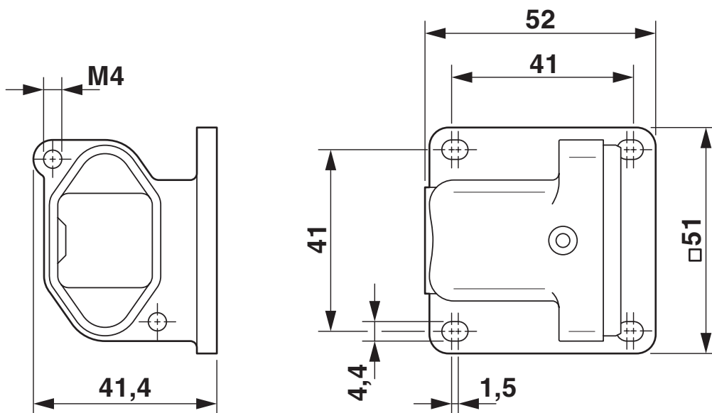
Maßzeichnung
