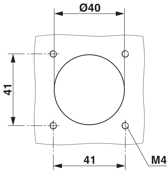
Dessin coté
