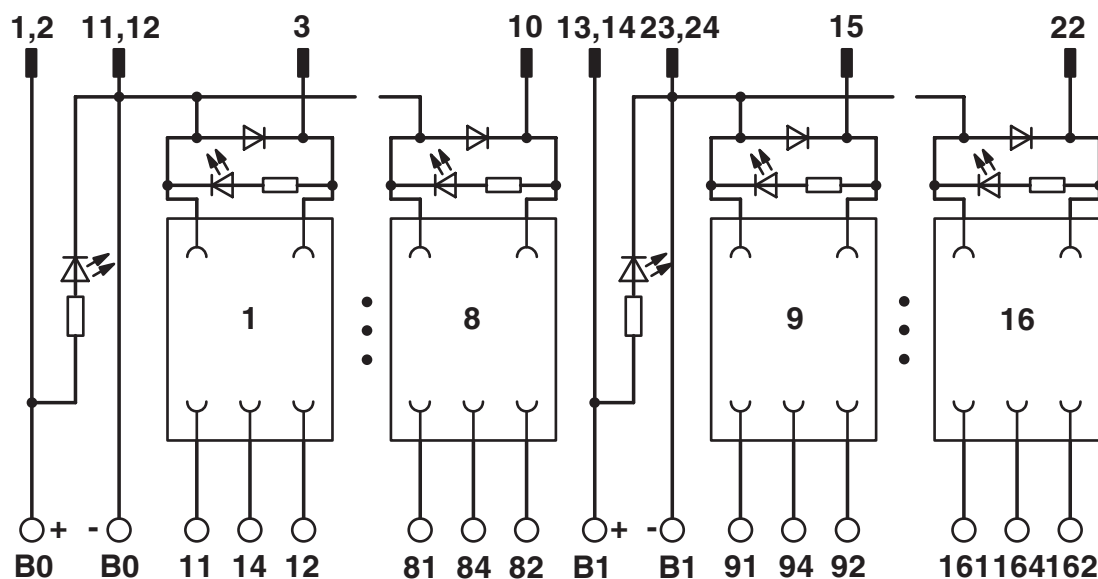
Diagrama eléctrico
