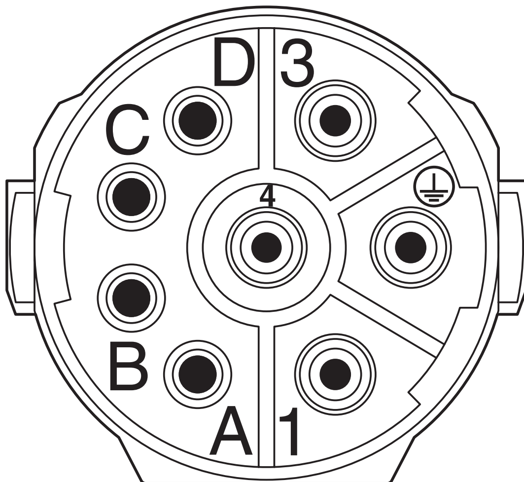
Dessin schématique
