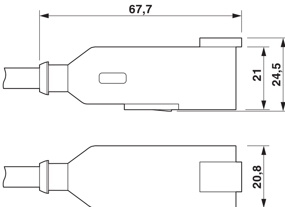
DEUTSCH DT04-6P, vista superior y lateral
