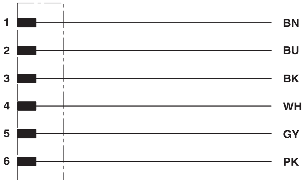
Diagrama eléctrico
