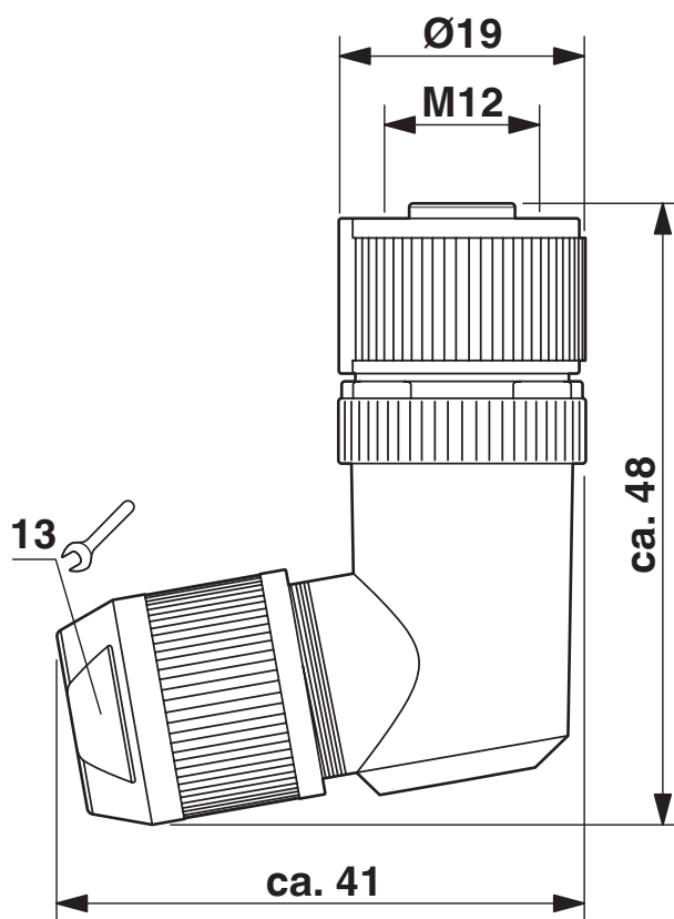
Conector hembra SPEEDCON M12, acodado, apantallado
