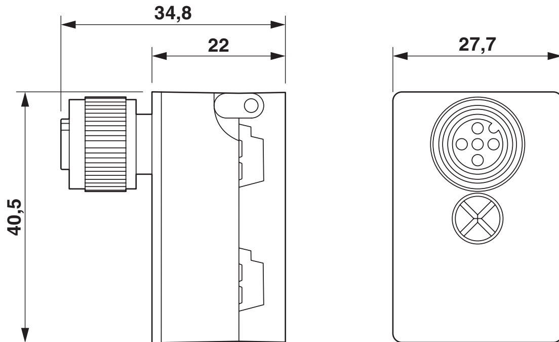
Verteiler, AS-Interface
