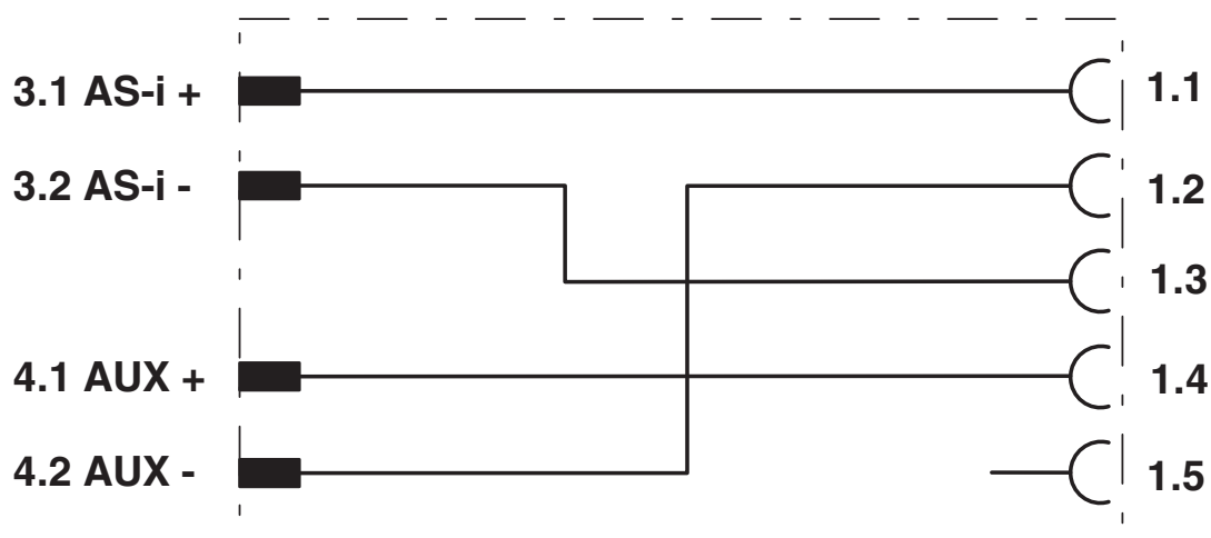
Schaltplan
