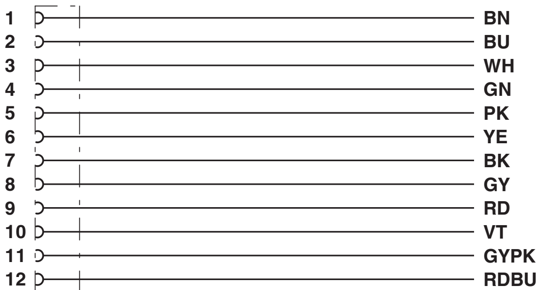
Ocupación de contactos del conector hembra M12
