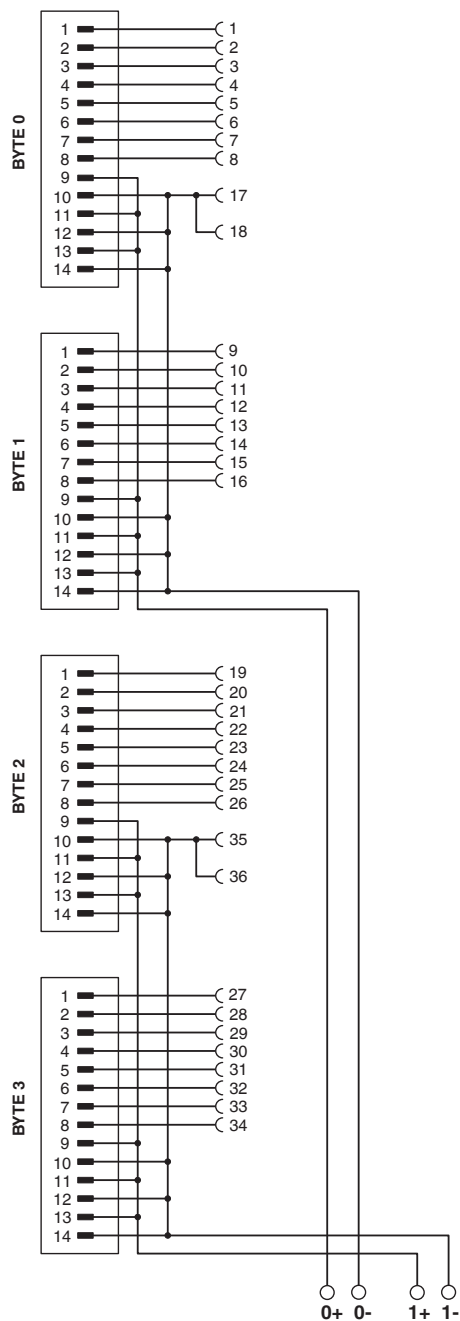
Schaltplan
