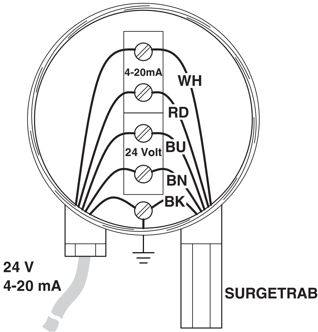
Applikationszeichnung
