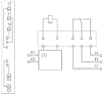
(1) Sicherheitsschaltung
