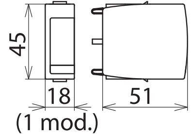
Maßbild DG PLU 550
