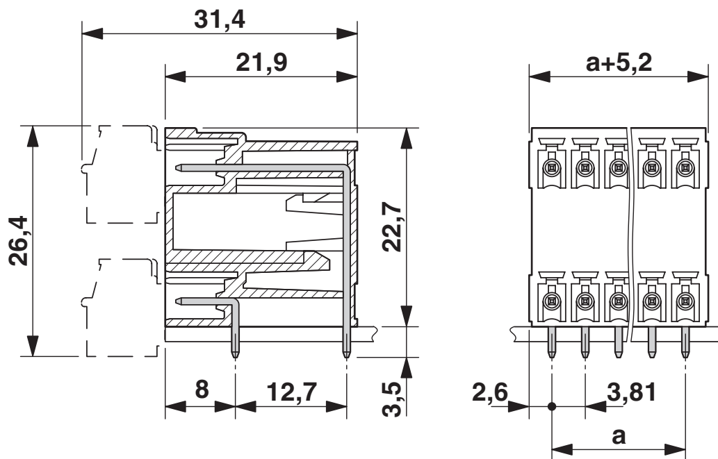
Maßzeichnung
