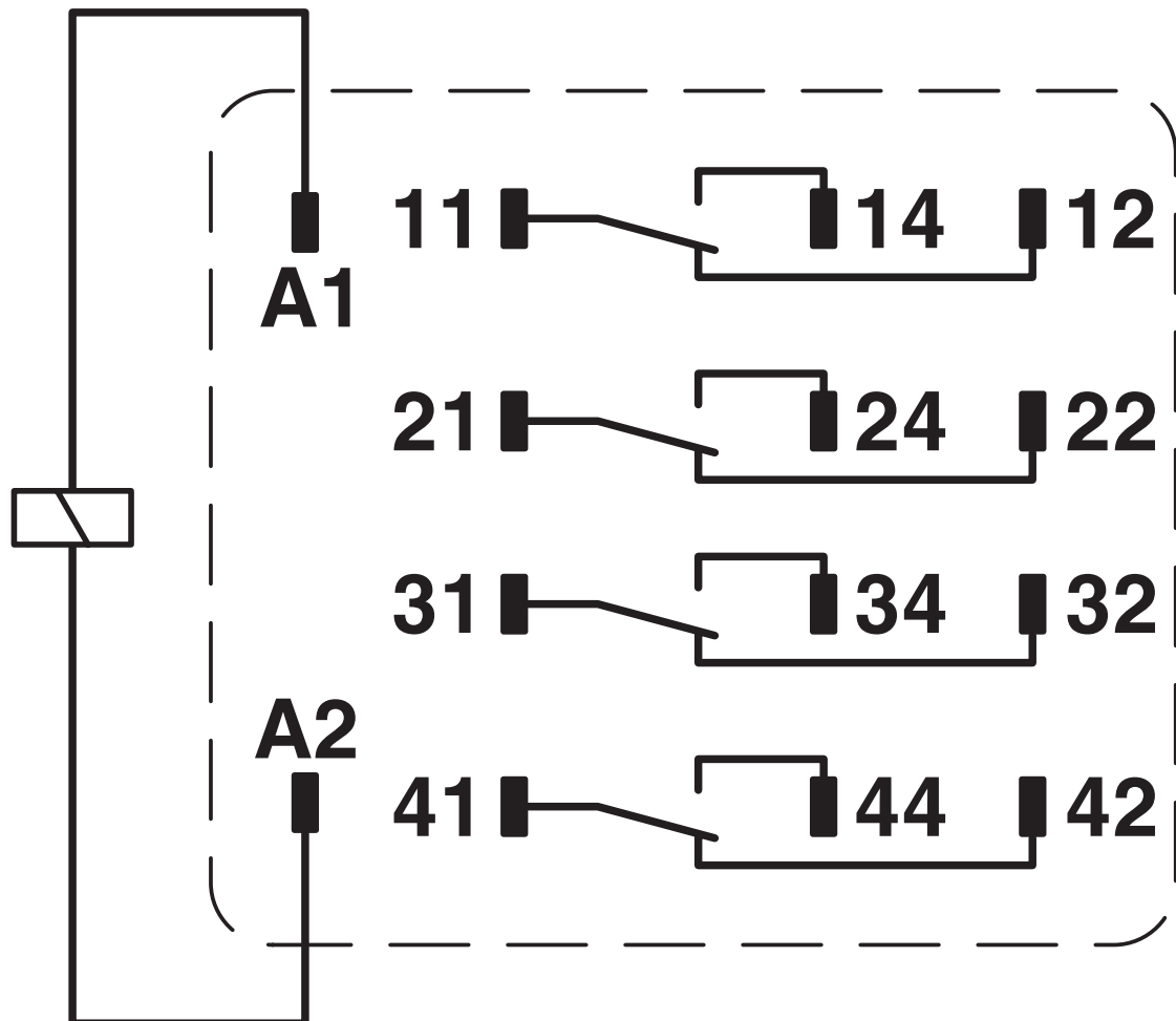
Diagrama eléctrico
