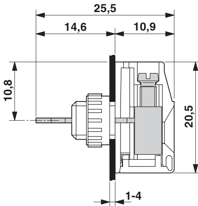
Dessin coté
