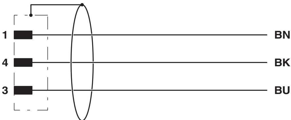
Diagrama eléctrico
