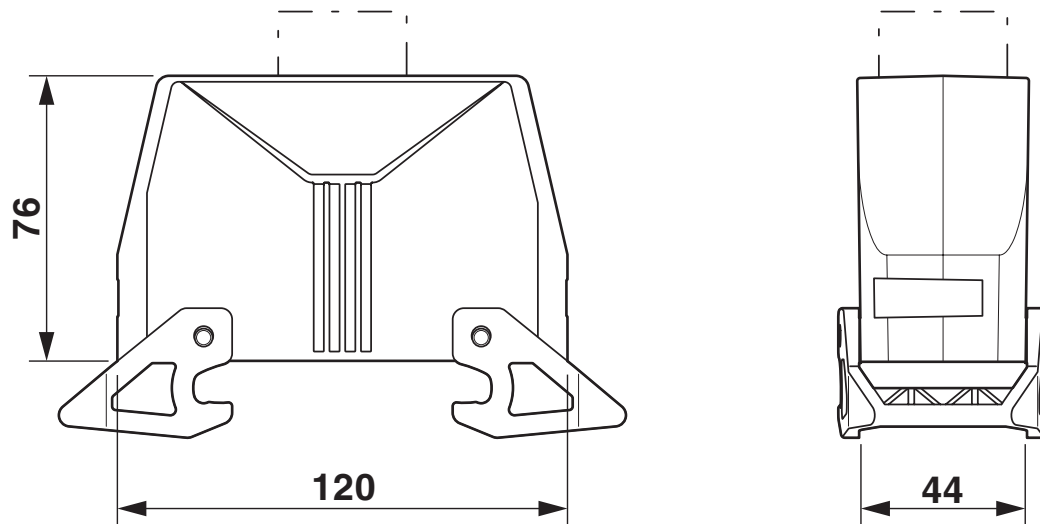
Maßzeichnung
