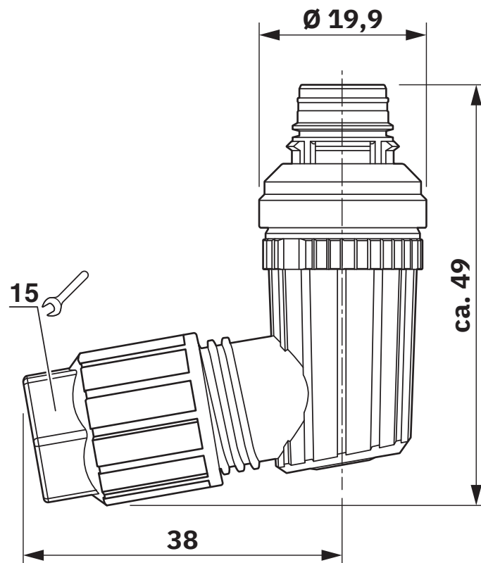
Maßzeichnung
