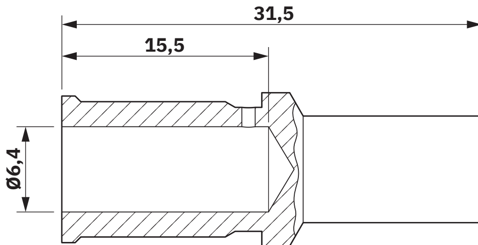
Maßzeichnung
