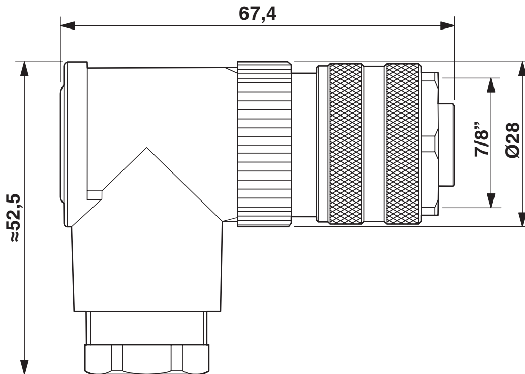
Maßzeichnung
