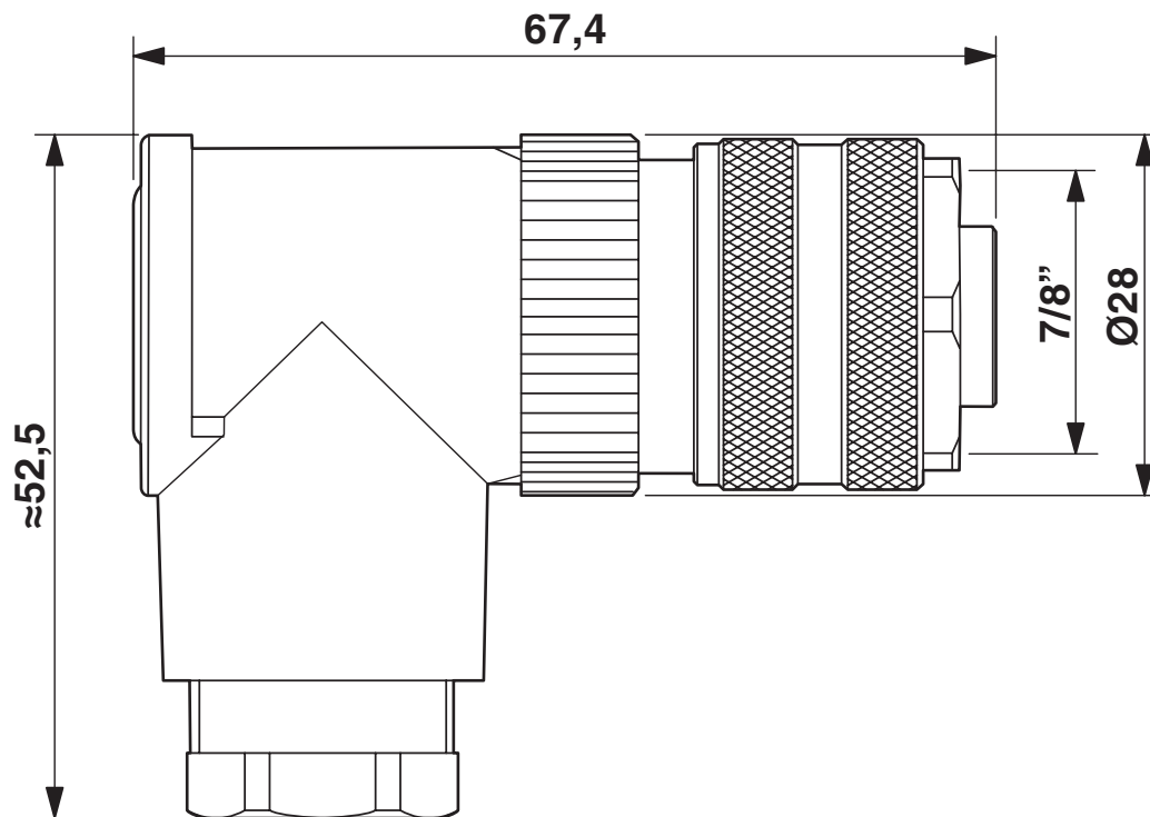
Dessin coté
