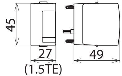
Maßbild DG MOD E DC 550
