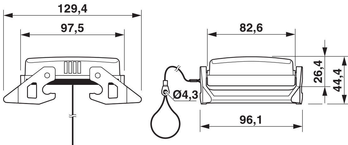
Dessin coté
