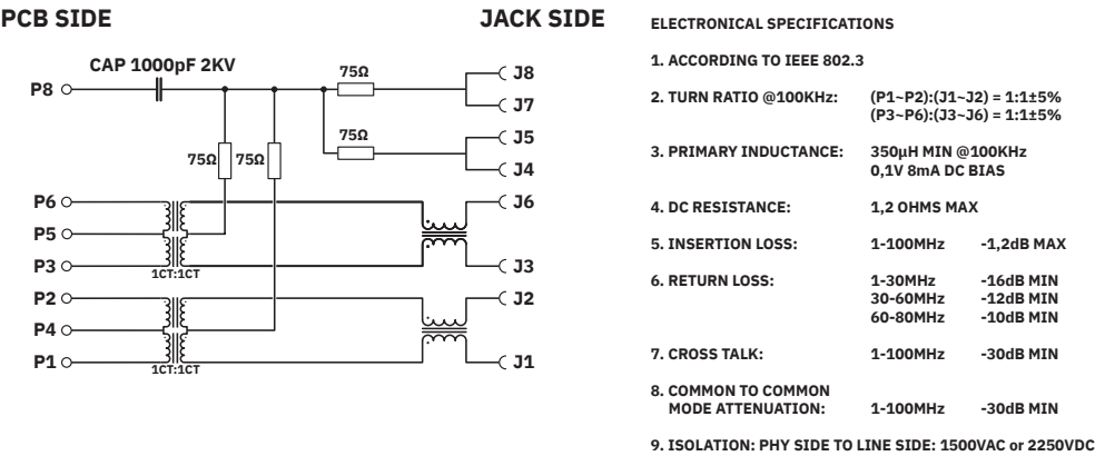
Diagrama eléctrico
