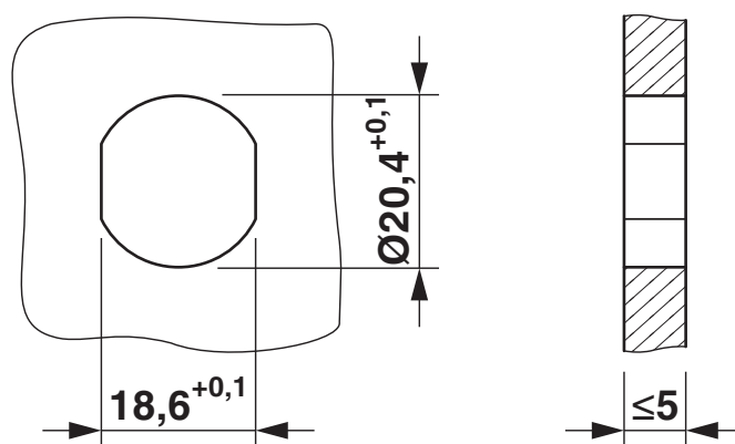
Gehäuseausschnitt für M20-Befestigungsgewinde, Montagewand mit Gewinde
