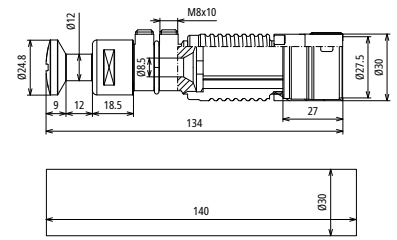
Maßbild AE ISO RIV KF HVI 90 V2A
