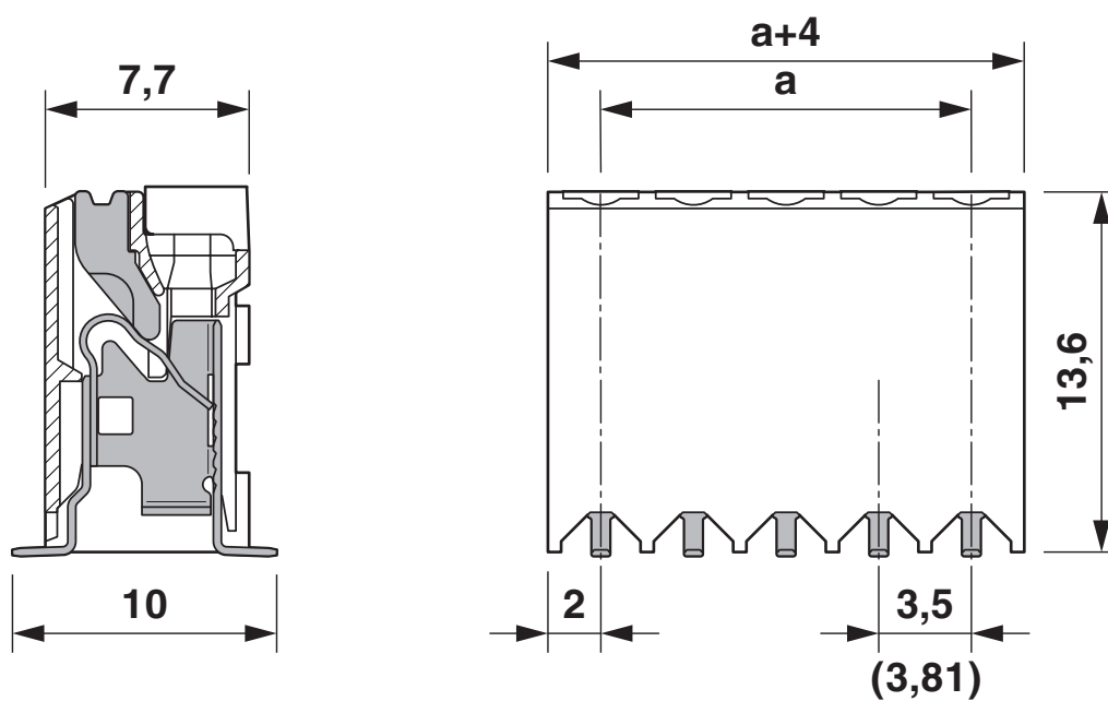
Maßzeichnung
