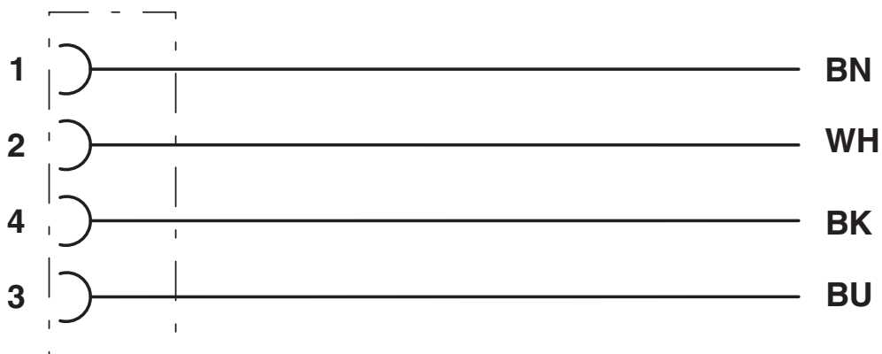
Ocupación de contactos del conector hembra M12
