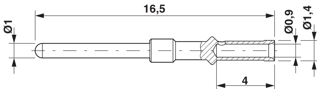
Dessin coté
