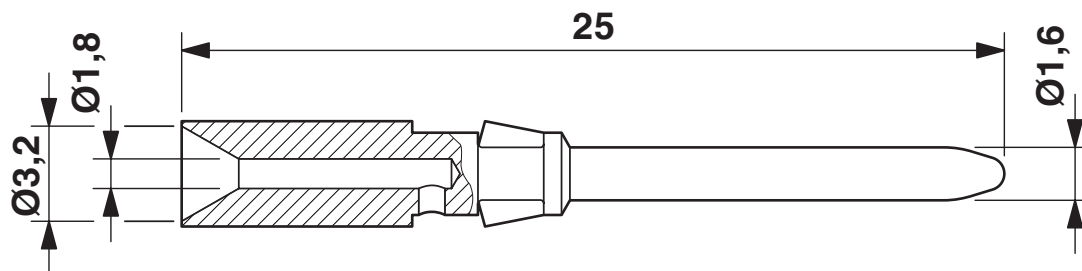
Dessin coté
