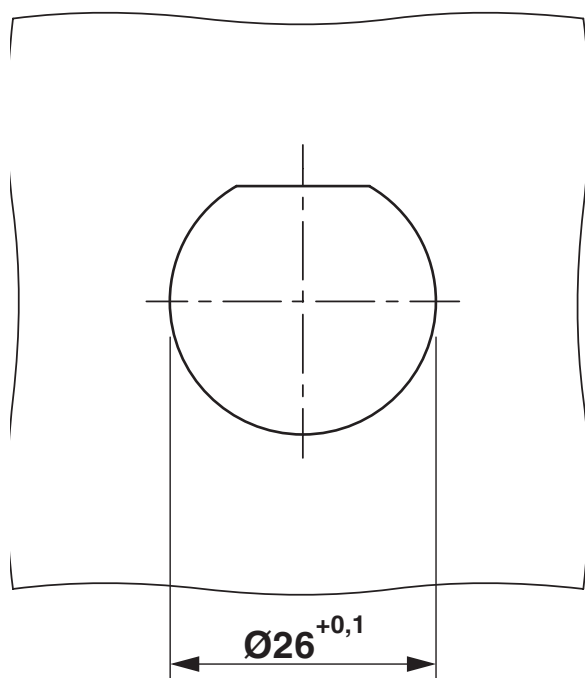
Maßzeichnung
