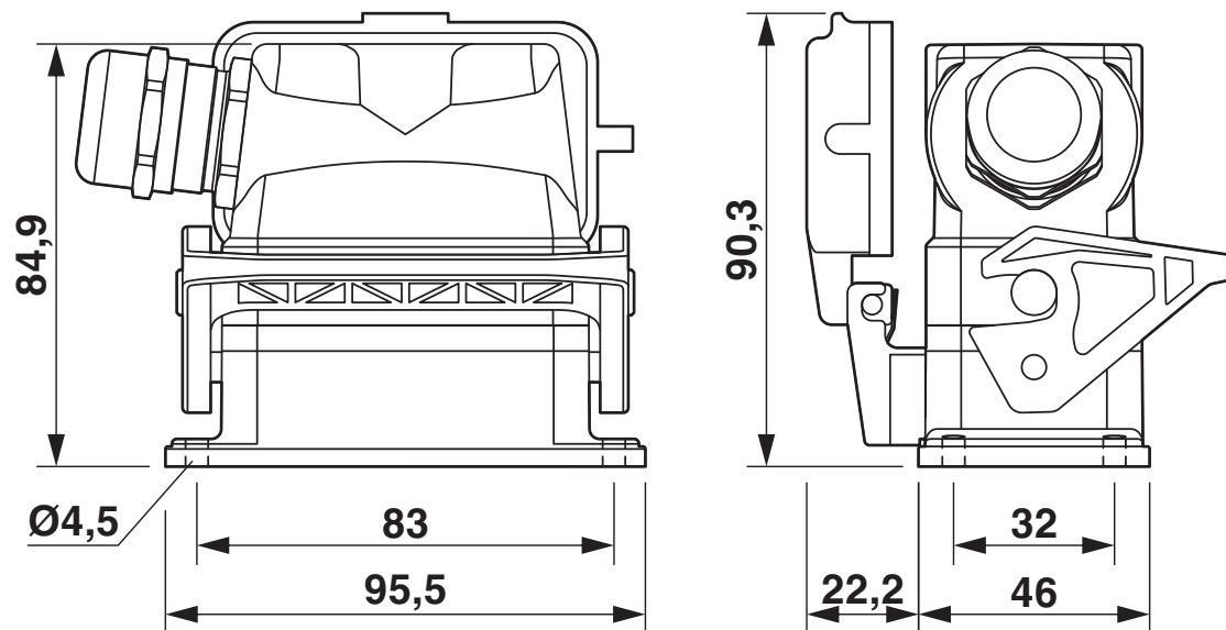
Maßzeichnung
