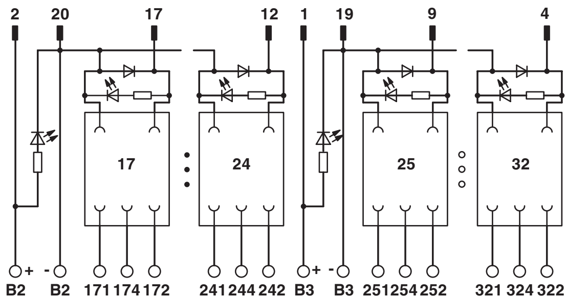
Schaltplan
