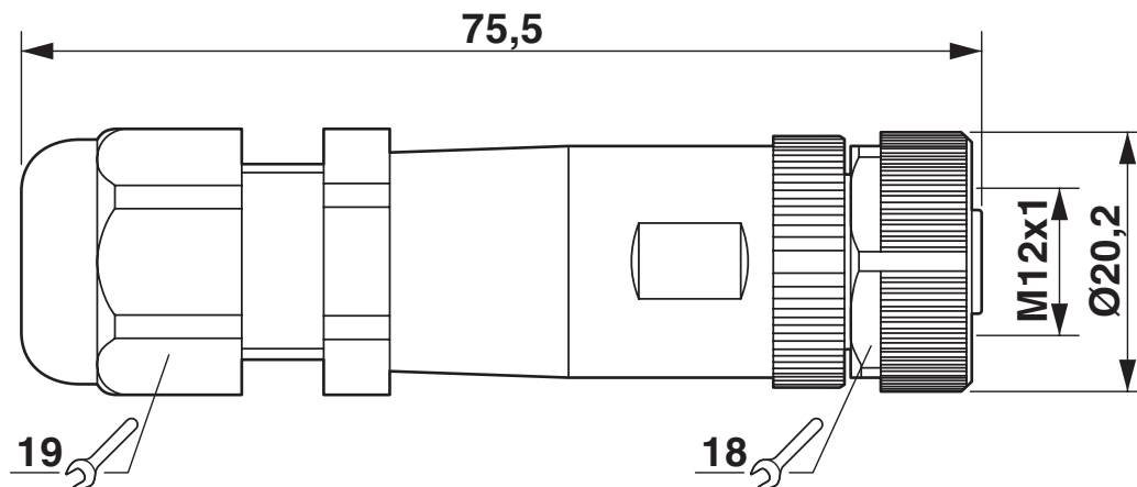
Maßzeichnung
