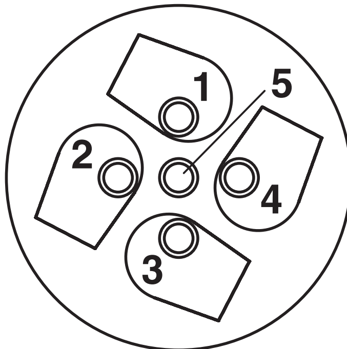
Schemazeichnung
