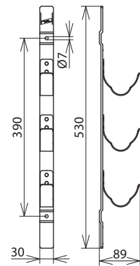
Maßbild HV 3HH ET
