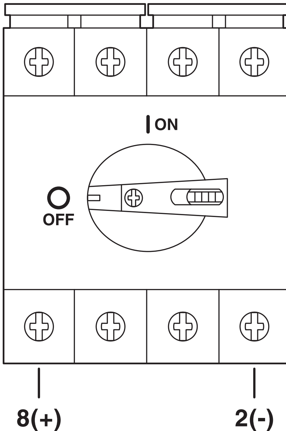
Dessin schématique
