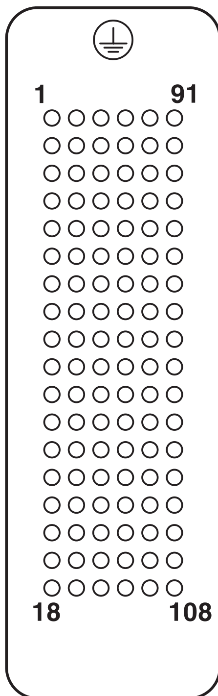
Dessin schématique
