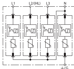
Prinzip Schaltbild DG MU 3PH 240 4W+G
