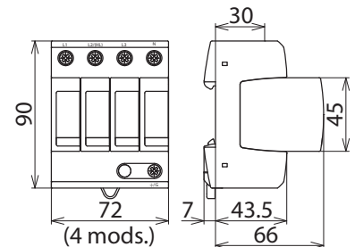
Maßbild DG MU 3PH 240 4W+G
