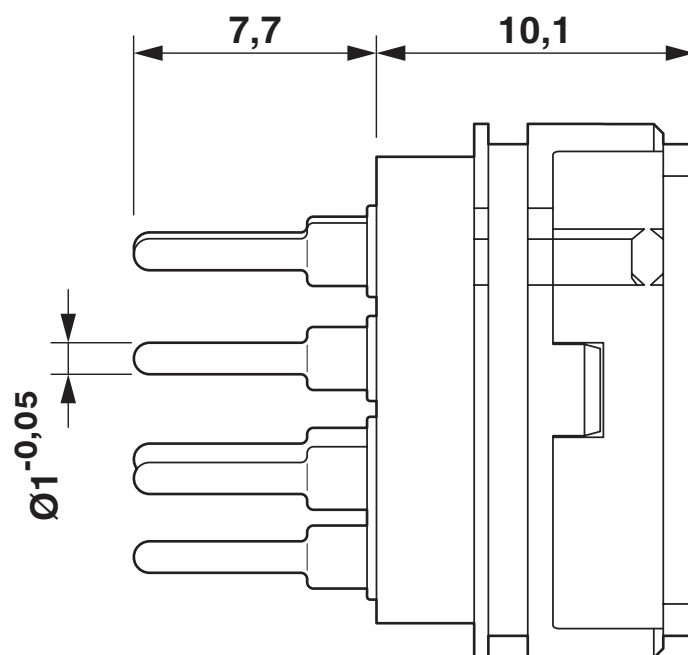
Dessin coté
