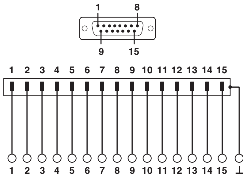
Schaltplan
