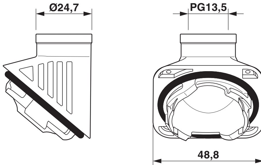
Maßzeichnung
