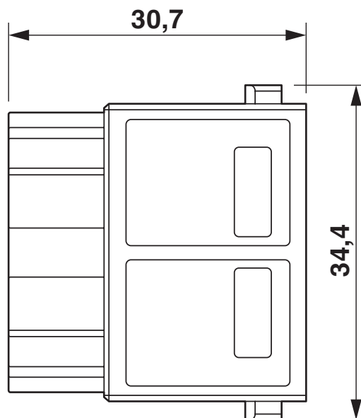
Dessin coté
