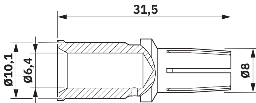
Dessin coté
